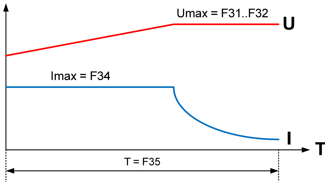
Рисунок 3.1 Диаграмма напряжений и токов в режиме ускоренного заряда
