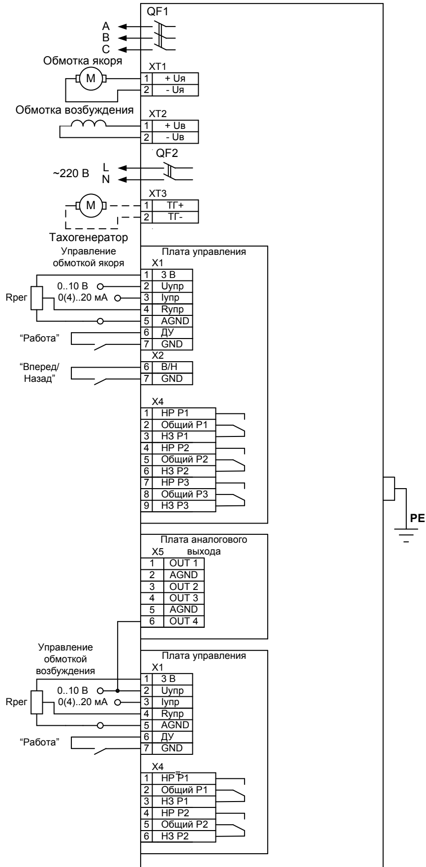
Рисунок А1 Схема подключения
