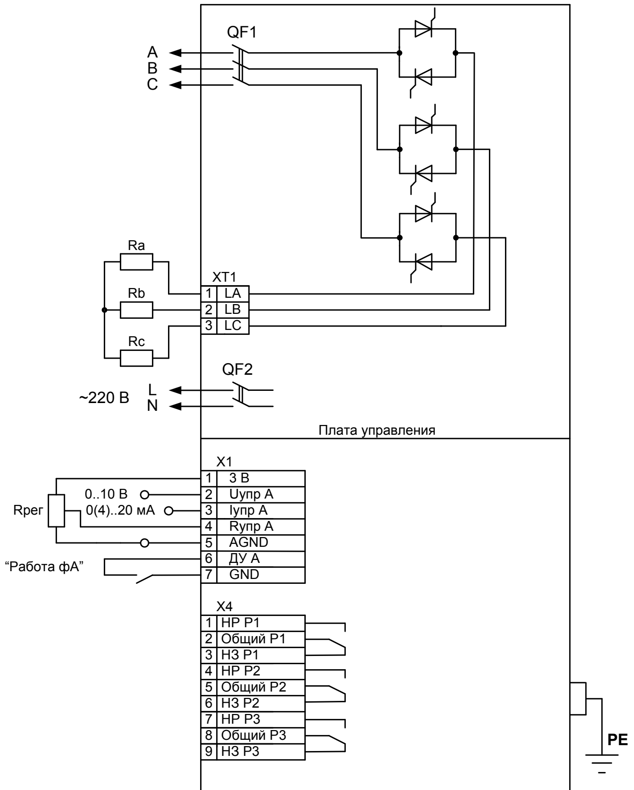
Рисунок А1 Схема подключения нагрузки – “звезда”
