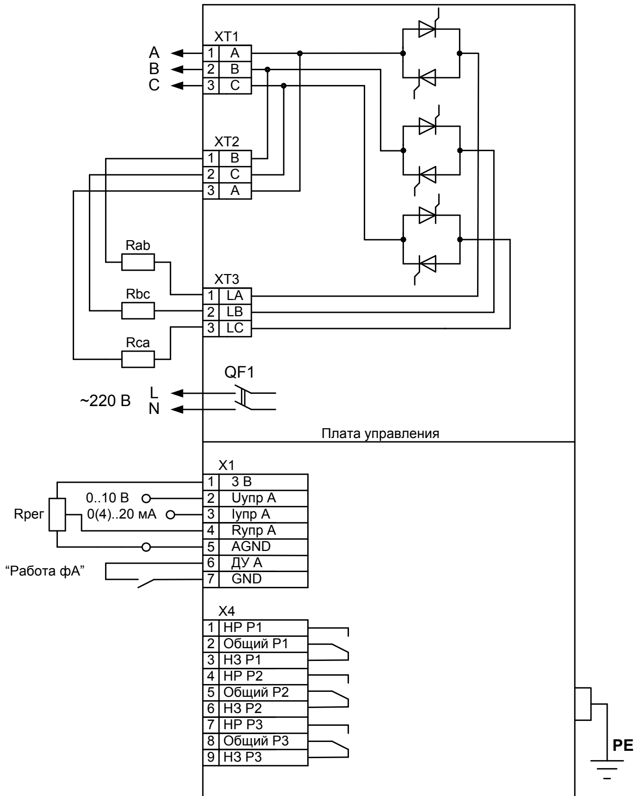
Рисунок А1 Схема подключения нагрузки – разомкнутый "треугольник"
