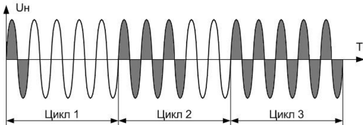
Рисунок 3.5 Выходное напряжение при регулировании методом пропуска периодов
