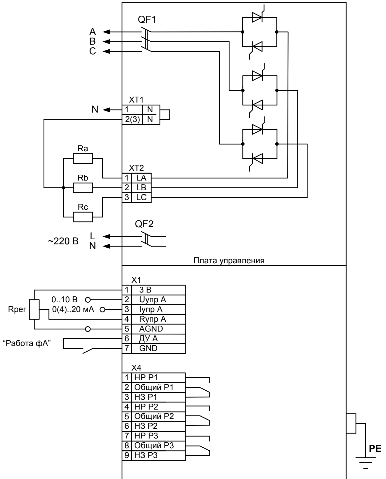
Рисунок А1 Схема подключения нагрузки – “звезда” с рабочей нейтралью
