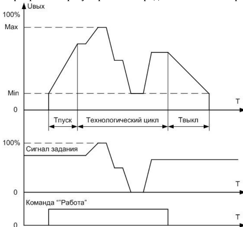
Рисунок 3.4 Рабочий цикл при фазовом методе регулирования
