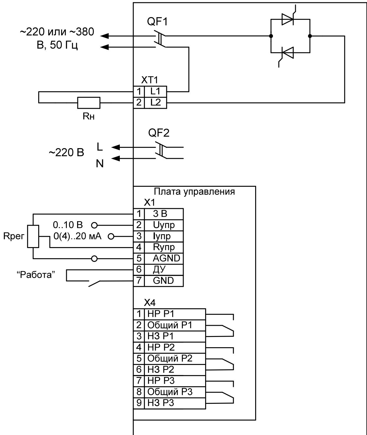
Рисунок А1 Схема подключения нагрузки
