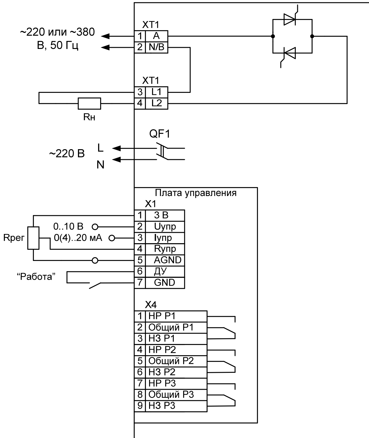
Рисунок А1 Схема подключения внешних проводов
